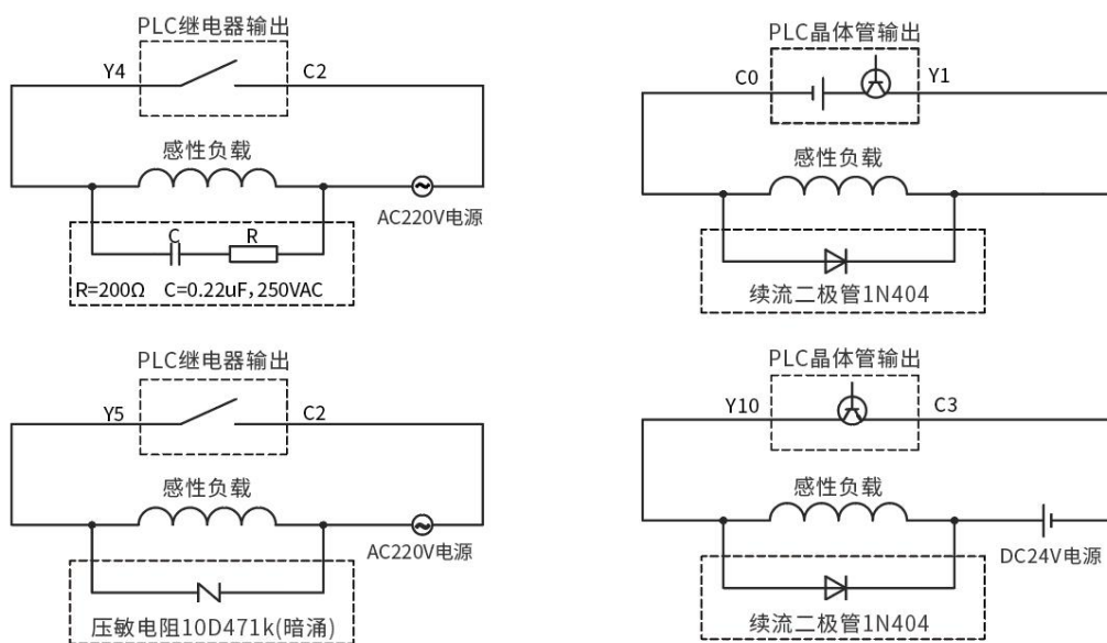
感性负载吸收电路示意图
