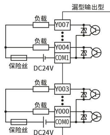
晶体管输出等效电路
