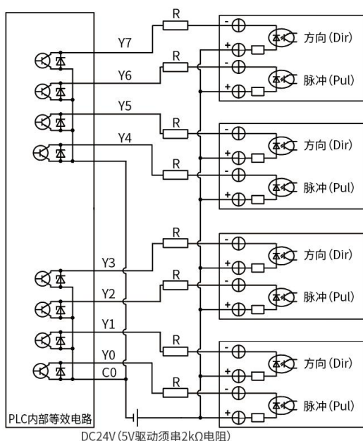
脉冲输出接线图
