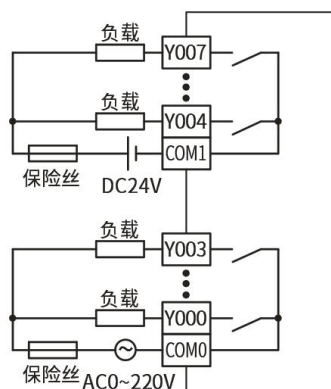
继电器输出等效电路
